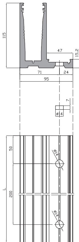
PERFIL U.L. 54301 MF-01
