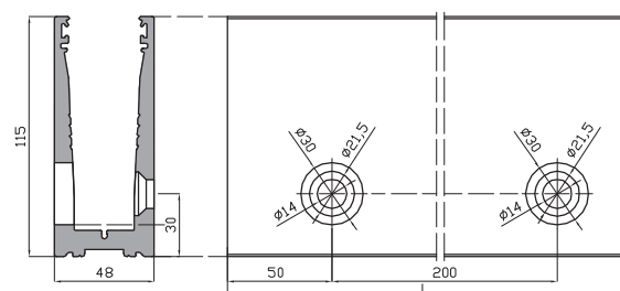
Pefil U 54300-MF03
