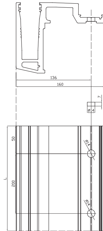
Perfil U.L. Frontal 54303-MF01
