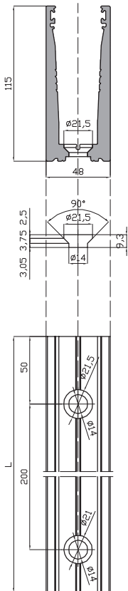
Pefil U 54300 MF-01
