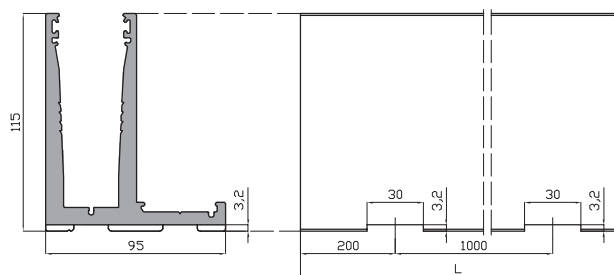
PERFIL U.L. 54301 MD-01
