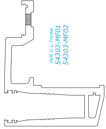
Mecanizado de Fijación Vertical
