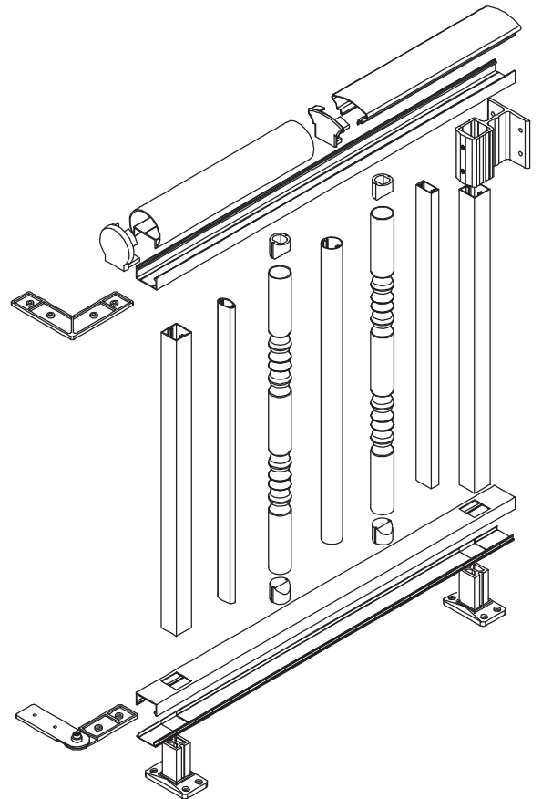
BARANDILLA CONVENCIONAL
